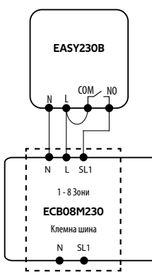
в) Схема на свързване към клемна шина
